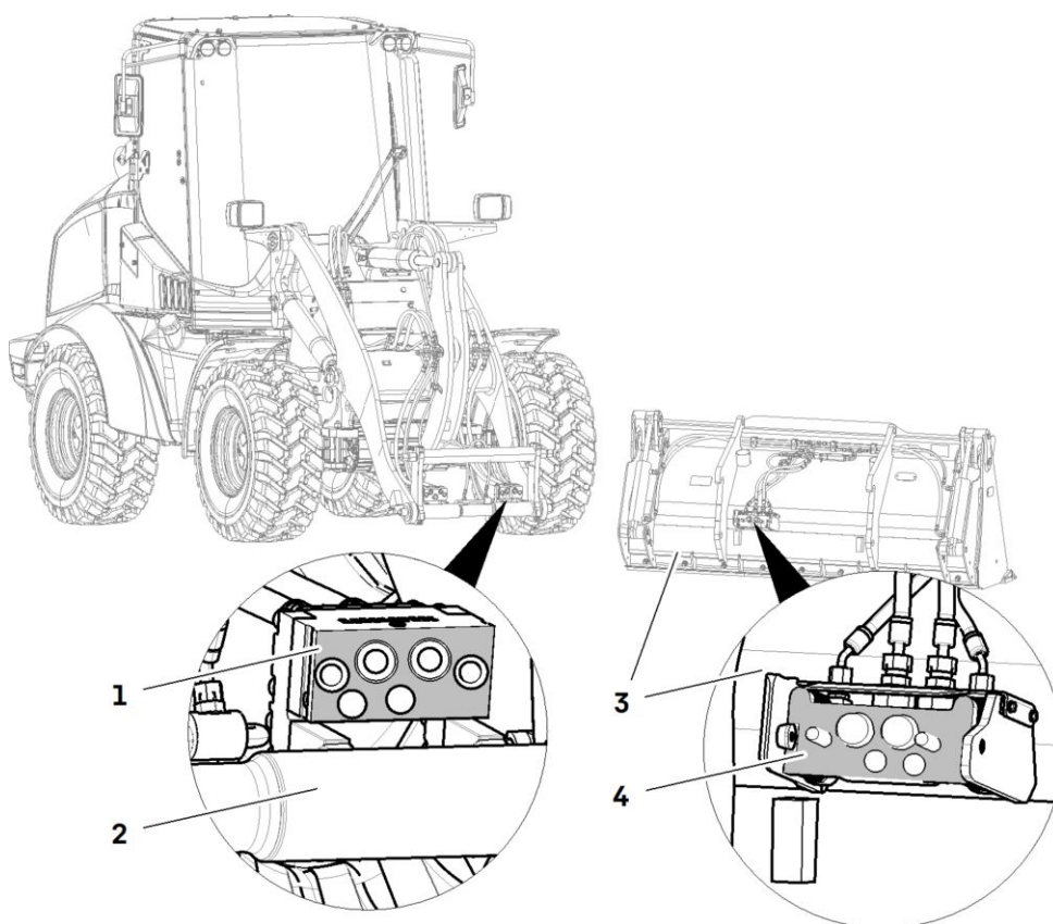
Attache rapide à système d'accouplement hydraulique « LIKUFIX »
