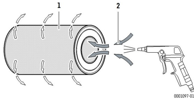
Nettoyage de l'élément filtrant principal
