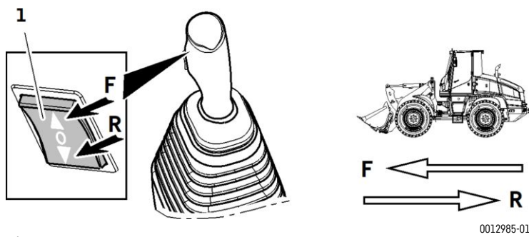
Sélectionner le sens de translation
