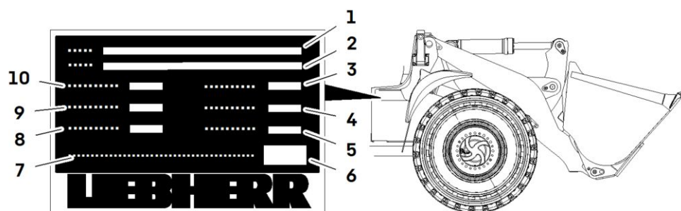
Plaque d'identification de la machine
