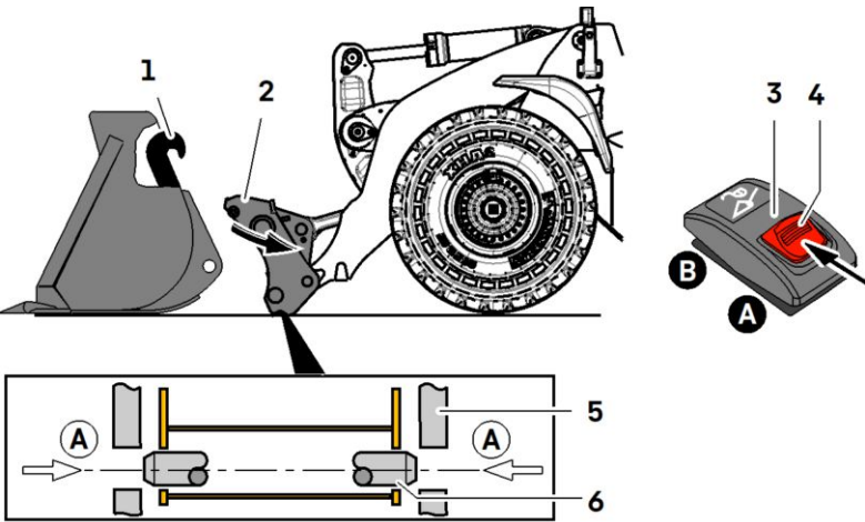
Déverrouillage et désaccouplement de l'équipement de travail
