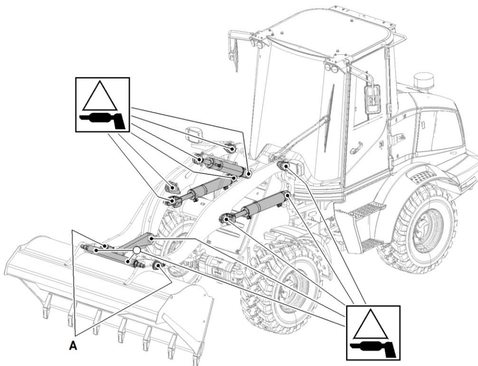
Graissage de bras de levage
