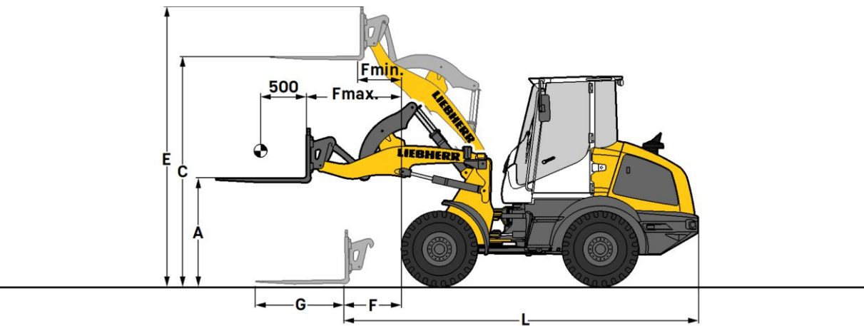
Équipement de travail « fourche FEM II »
