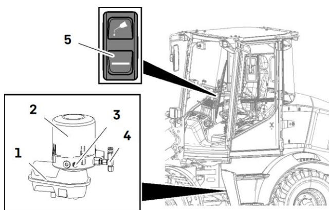
Circuit de graissage centralisé
