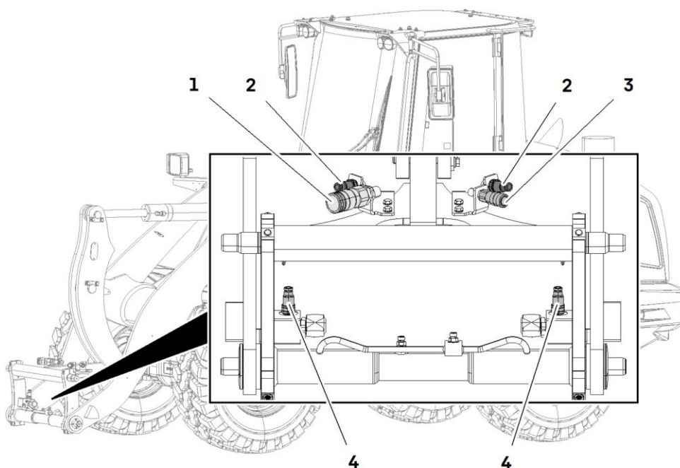
Raccords hydrauliques pour équipements de travail hydrauliques
