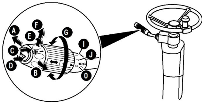
Commutateur de colonne de direction
