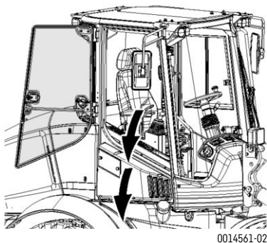
Sortir de la cabine par la sortie de secours
