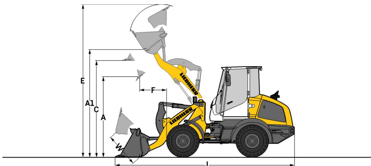
Équipement de travail « godet 4-en-1 »
