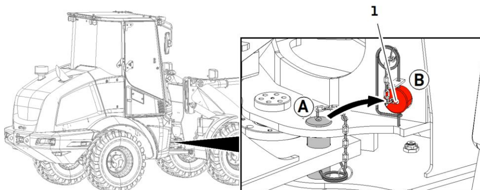
Débloccage de l'articulation
