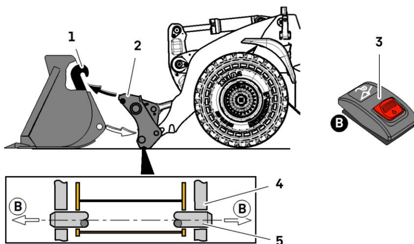
Accouplement et verrouillage d'un équipement de travail
