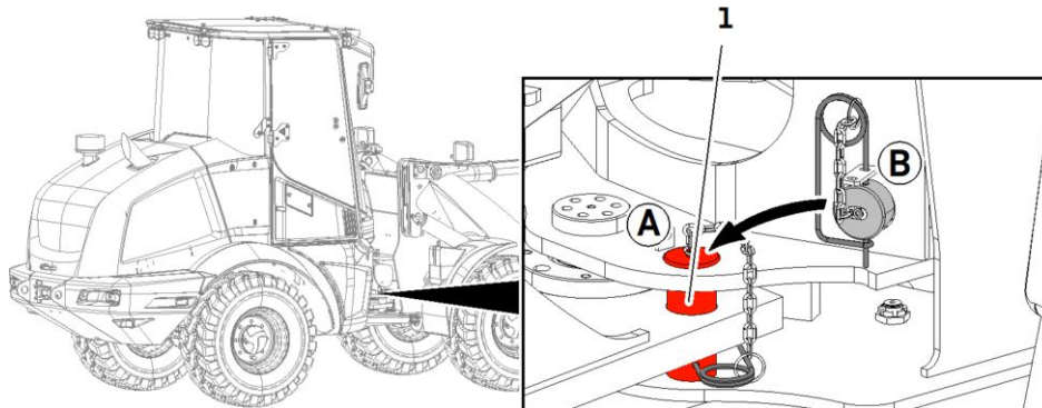
Enclenchement du blocage d'articulation
