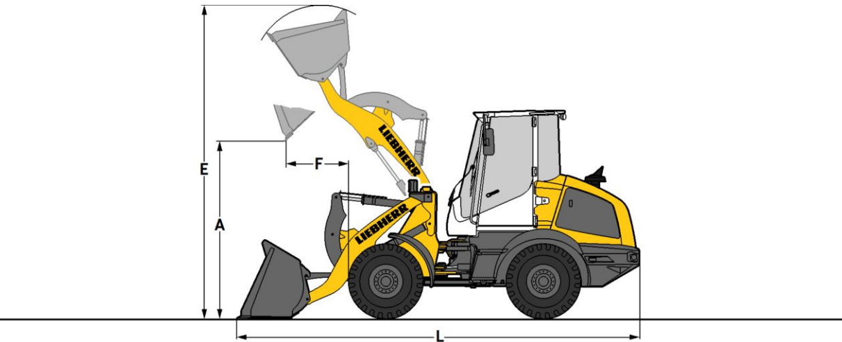
Équipement de travail « godet pour matériaux légers »
