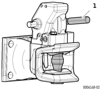
Désaccouplement de la remorque
