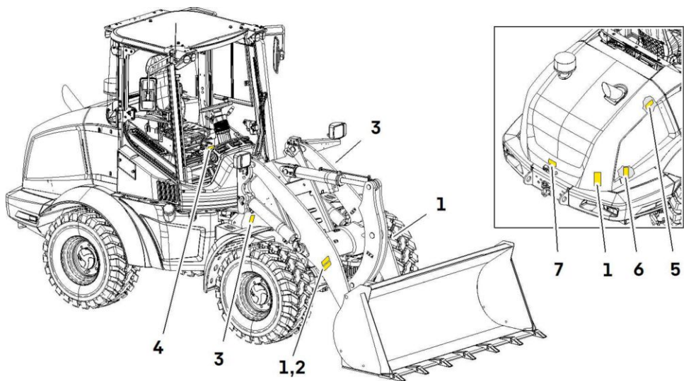
Disposition des plaques de sécurité
