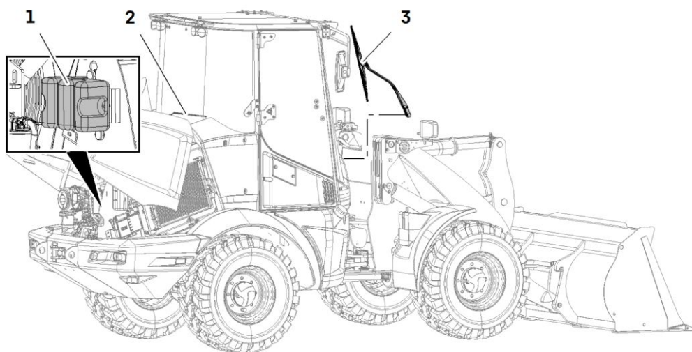
Dispositif de lave-glace
