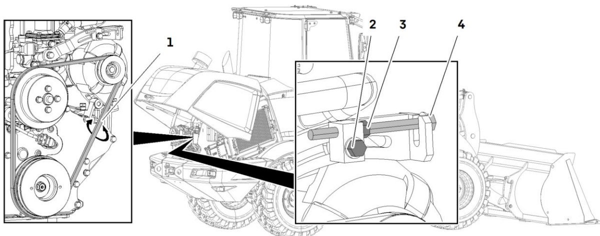
Contrôle de la courroie trapézoïdale du moteur Diesel
