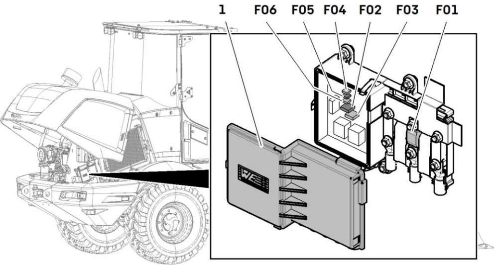
Fusibles du compartiment moteur droit
