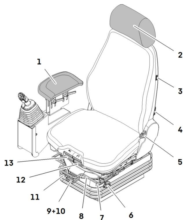
Siège « Grammer Confort »
