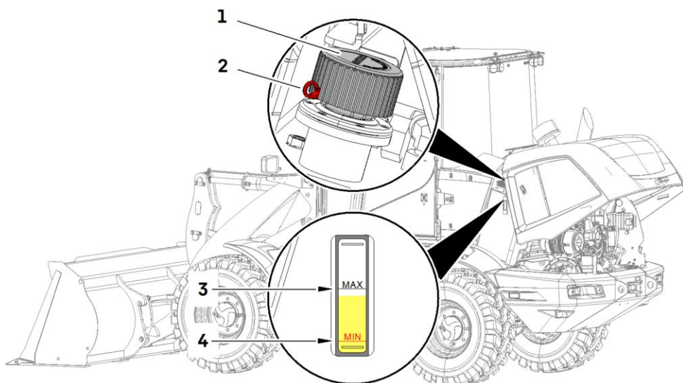
Contrôle de niveau d'huile
