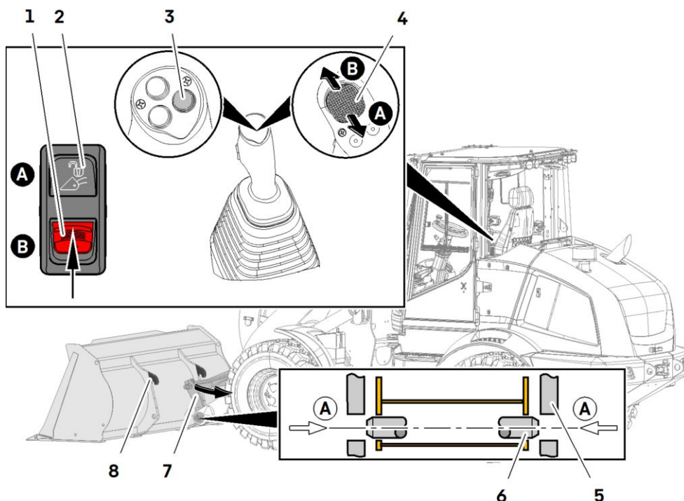
Déverrouillage et désaccouplement de l'équipement de travail
