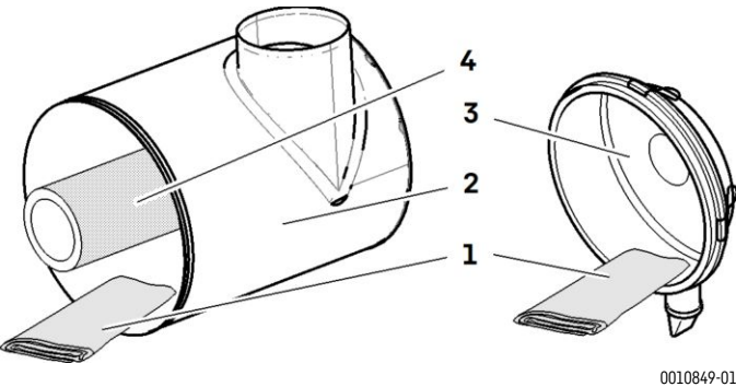
Nettoyage du couvercle de service et du carter de filtre
