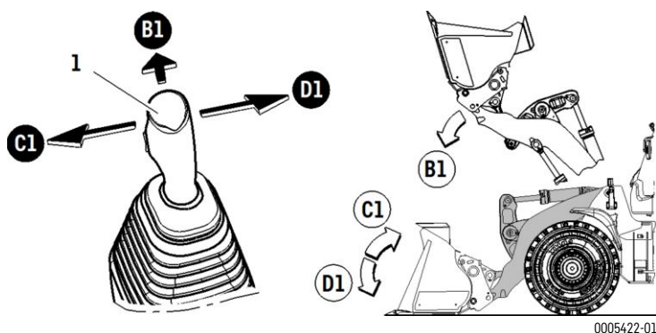
Abaissement de l'équipement de travail
