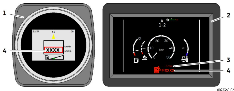
Dispositif de protection contre les sursrégimes
