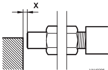
La distance (X) entre le bras de levage et le capteur doit être dans la plage 3–5 mm.
