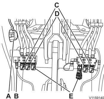
Figure illustrant toutes les options hydrauliques possibles
