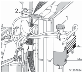
Vase d'expansion
