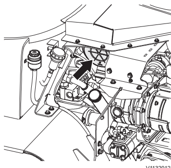
Filtre à air du moteur
