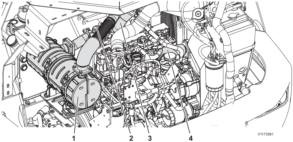
Surfaces chaudes dans le compartiment moteur (moteur D3.3M)
