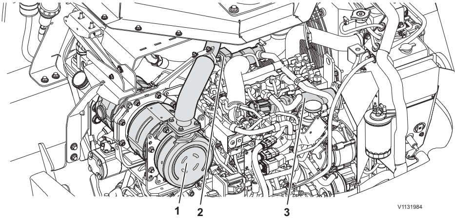
Surfaces chaudes dans le compartiment moteur (moteur D3.3H)
