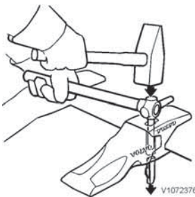
Extraire le dispositif de verrouillage
