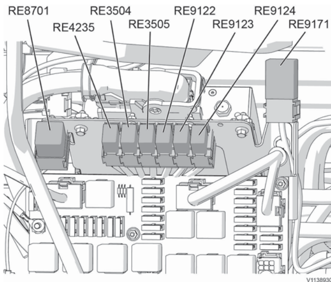
Support de relais au-dessus de la carte, module électrique central (ancienne version)
