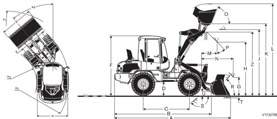
L35G avec tringlerie à barre en Z, porte-outils en Z et pneus 405/70 R20
