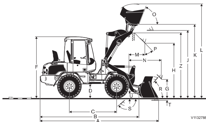
L35G avec tringlerie à barre en Z, porte-outils en Z et pneus 405/70 R20
