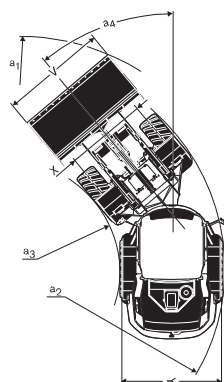
L35G avec tringlerie à barre en Z, porte-outils en Z et pneus 405/70 R20
