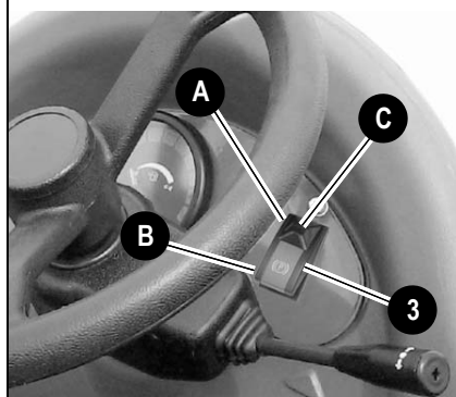
Fig. 35 : Frein de stationnement 1001/1501 (représentation symbolique)
