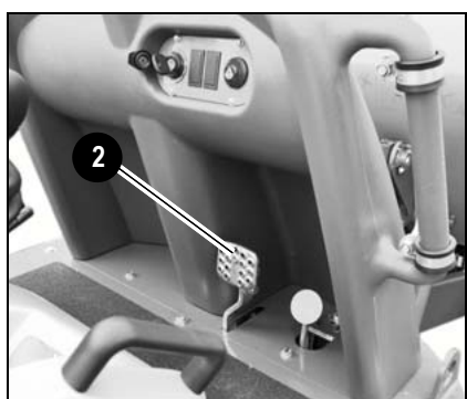
Fig. 33 : Pédale du frein 1001/1501
