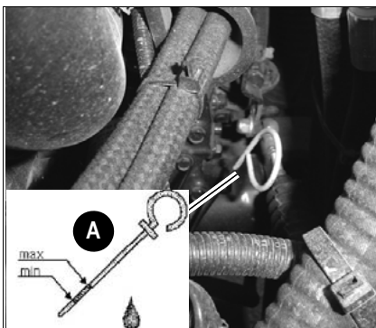
Fig. 80 : Contrôle du niveau d'huile
