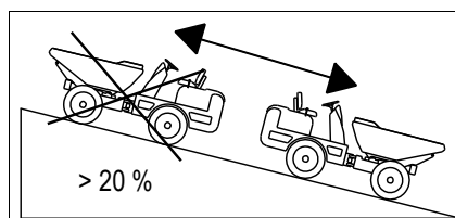
Fig. 40 : Conduite en pente sans charge
