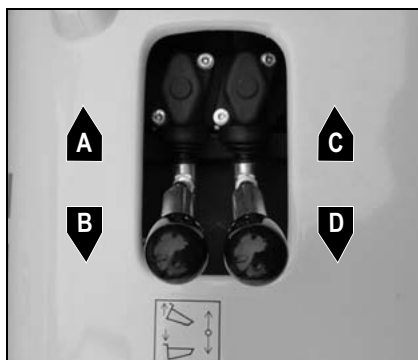
Fig. 49 : Commande de la benne rotative (1501S)
