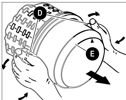
Fig. 84 : Dépose de la partie inférieure du boîtier
